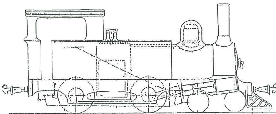
Automotor Berliet utilitzat a partir del 1926. Escala 1:75 (autor: Nicolau Cañellas)
