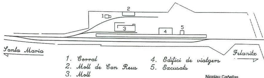
Cròquis de l'estació de Porreres (autor Nicolau Cañellas)
